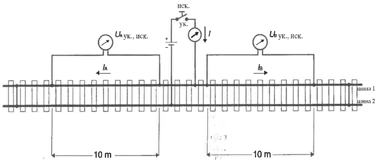
Slika 5.1. Određivanje otpora šine dužine 10m
