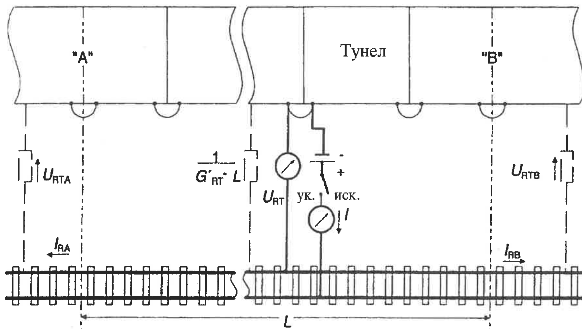
Slika 5.2.: Određivanje podužne odvodnosti G'_{RT} između voznih šina i tunela
